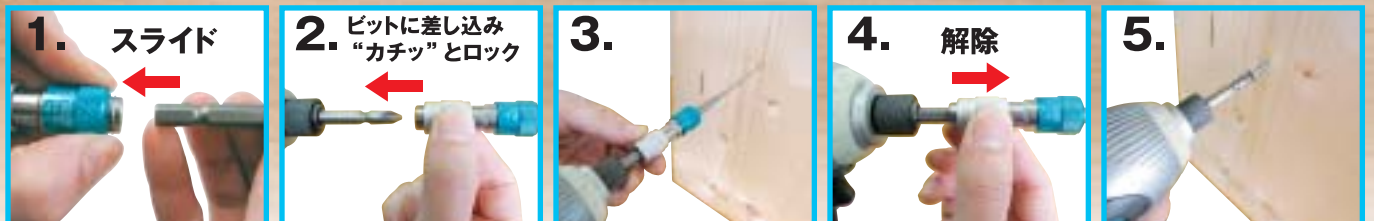
1. スライド 下穴錐を装着する。 2. ビットに差し込み "カチッ" とロック ホワイト側ローレットを持ってドライビットに装着する。 3. (Drilling) 下穴錐で穴あけ作業 4. 解除 ホワイト側ローレットを持ってビットジョイントを取り外す。 5. (Drilling) ドライビットでネジ締め作業
